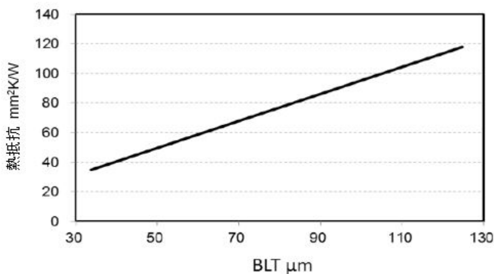
図 TIG1500の厚み (um)と熱抵抗の関係 (mm²K/W)
